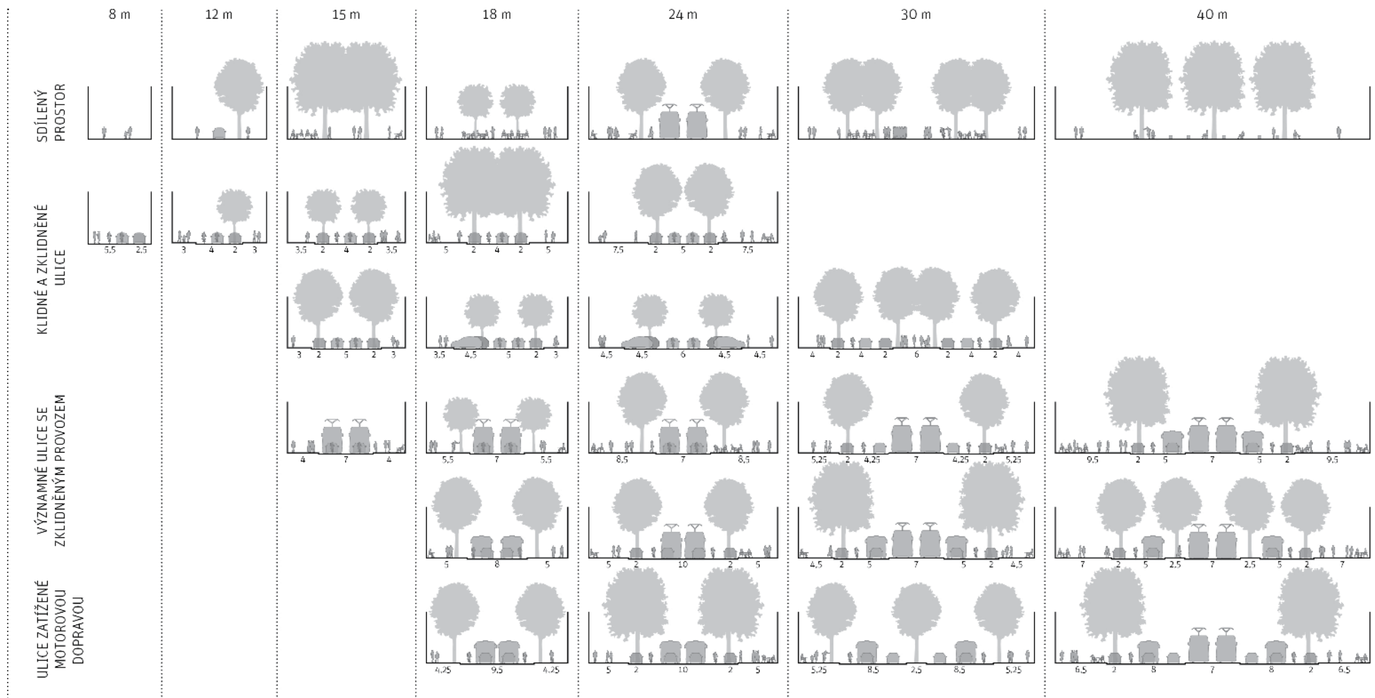
so4 PŘÍKLADY ULIČNÍCH PROFILŮ A CHARAKTERŮ JEJICH PROVOZNIHO USPOŘÁDÁNÍ Tabulka představuje ukázky možných řešení uspořádání uličních profilů v závislosti na šířce ulice.
