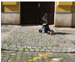
090 Napojení vjezdu na vozovku nenarušuje kontinuitu chodníku ani komfort a bezpečnost chůze [ Praha 7, Bubeneč ]
