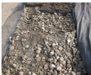
322 Strukturální zemina brání zhutnění a zajišťuje přístup kyslíku. Přitom umožňuje pokládání dlažby podobně jako na rostlý terén
