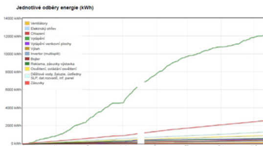
Elektrické vytápění činilo podstatnou část spotřeby energie v topném období a podílelo se na celkové spotřebě 59, 8 %.
