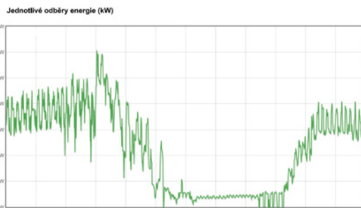
Z tohoto grafu záznamujícího spotřebu energie na vytápění je vidět zásadní vliv tepelných zisků (slunce-šlátech) na spotřebě energie. K průměru využití tohoto efektu je však nezbytný šetrnější topný systém, schopný rychlé reakce a to v každém vytápěném prostoru samostatně. Klasické toplovodní systémy (s jakýmkoliv zdrojem) tuto schopnost v rZEB nemají.
